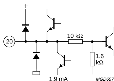
Fig.30 Pin 20; V_{OQSS} .
