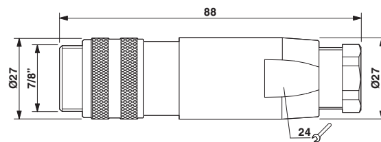
外形寸法
