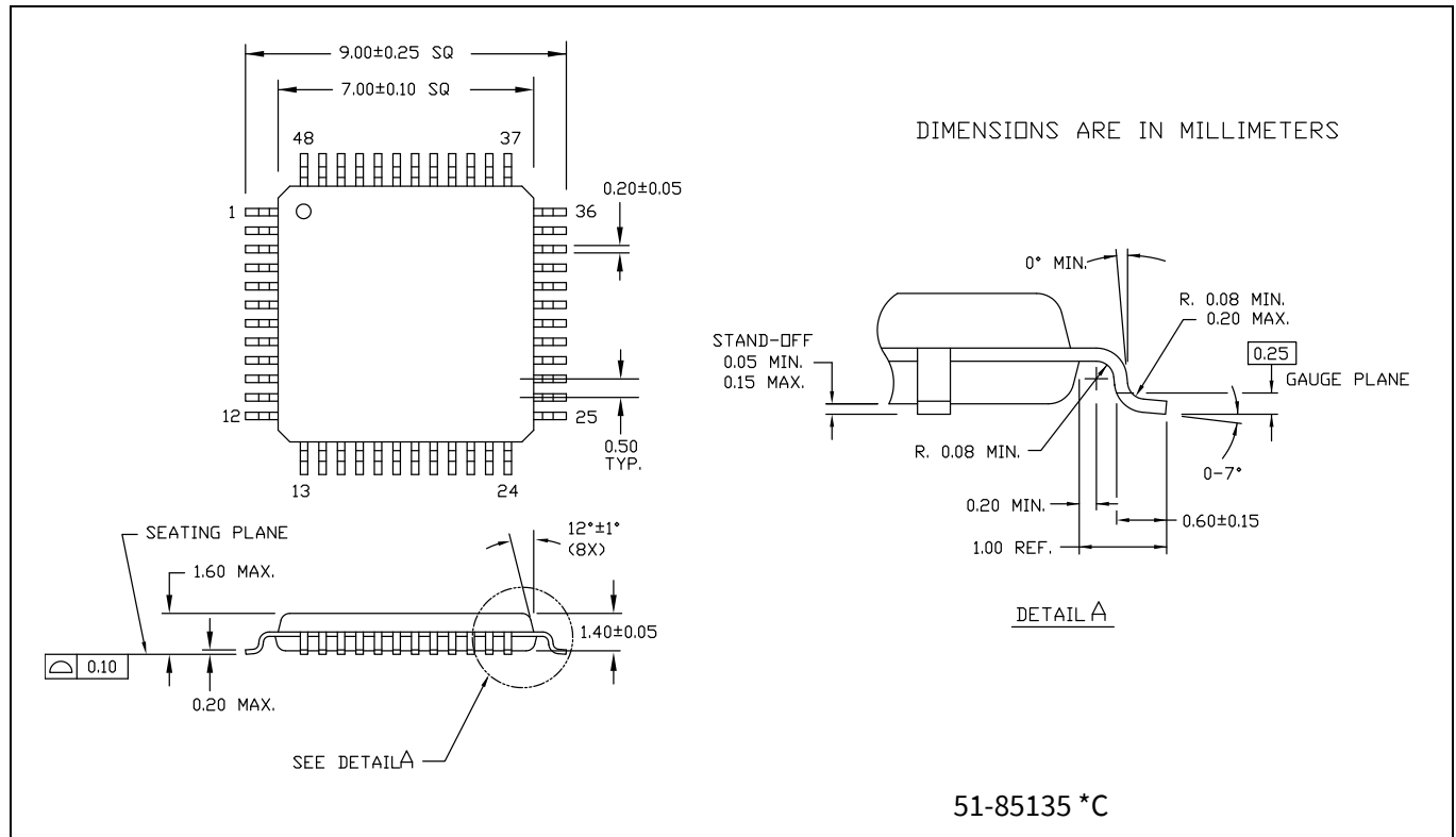
Figure 6 48LD TQFP 7×7×1.4 mm, パッケージ外形, (PG-TQFP-48)
