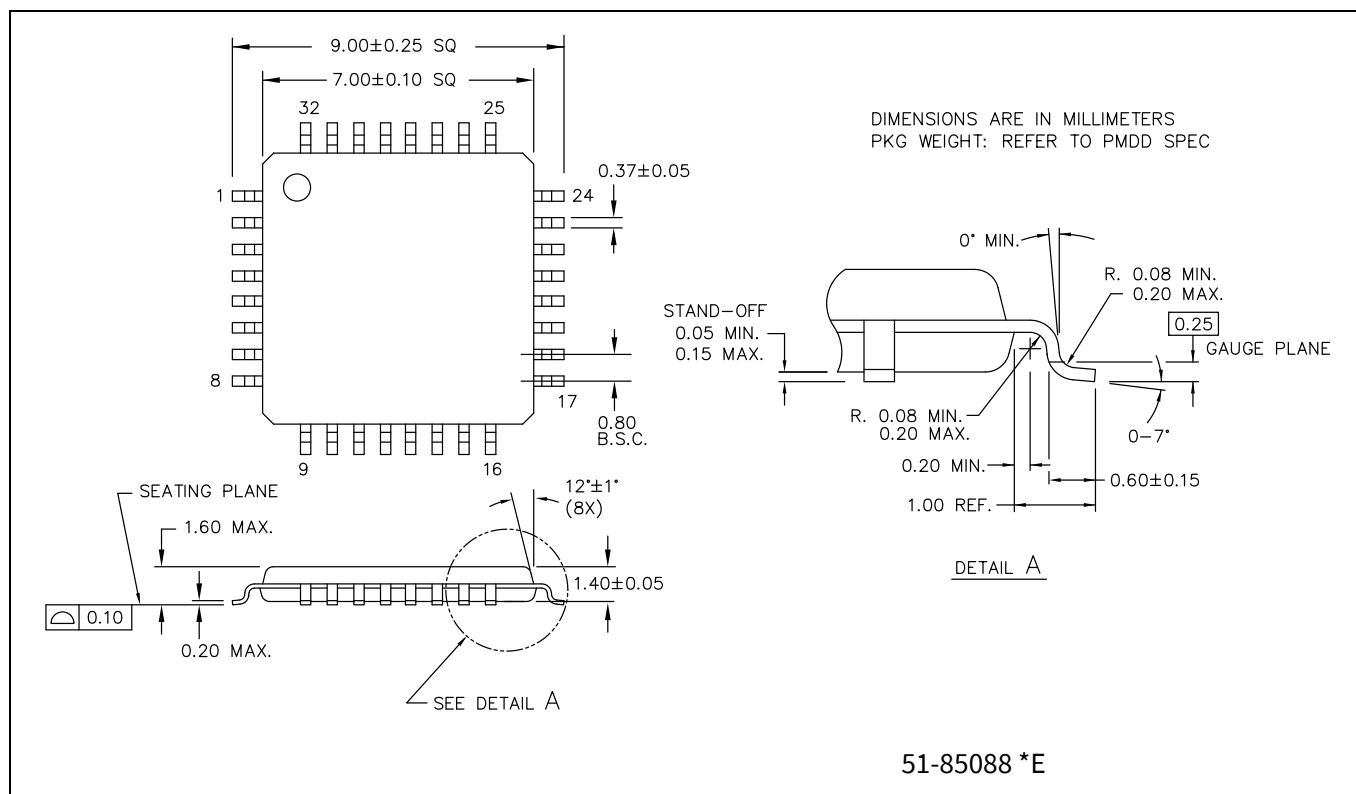
Figure 10 32LD TQFP 7×7×1.4 mm A3214, パッケージ外形, (PG-TQFP-32)
