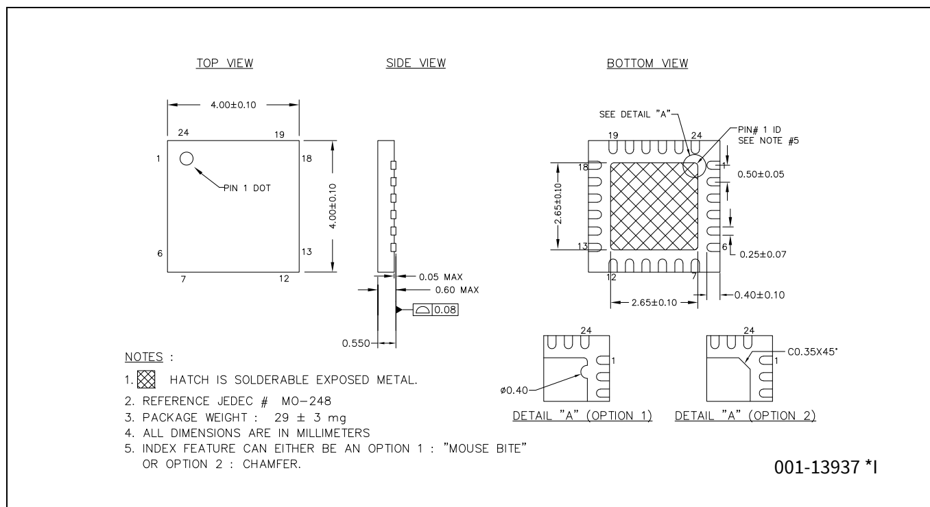
Figure 9 24L QFN 4×4×0.60 mm LQ24A/LQ24B 2.65×2.65 EPAD (SAWN), パッケージ外形, (PG-VQFN-24)
