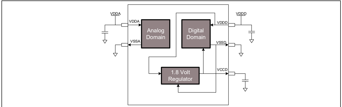
Figure 4 電源接続
