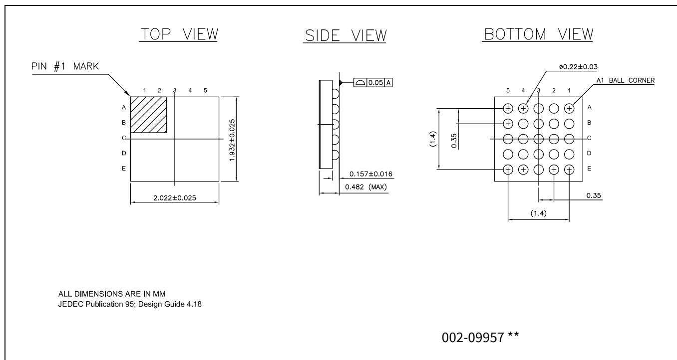
Figure 11 PSOC™ 4A S1 WLCSP 2.02×1.93×0.48 mm, パッケージ外形, (PG-XFWL-25)
