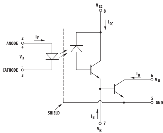
HCPL-270L/HCPL-070L
