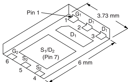
PowerPAIR® 6 x 3.7
