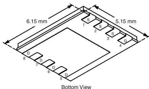
PowerPAK SO-8
