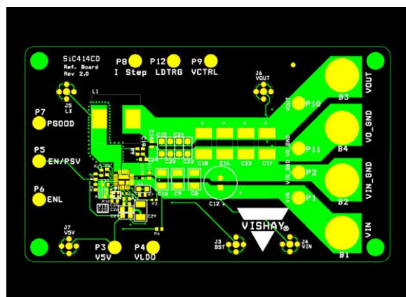
Fig. 14 - Top Layer
