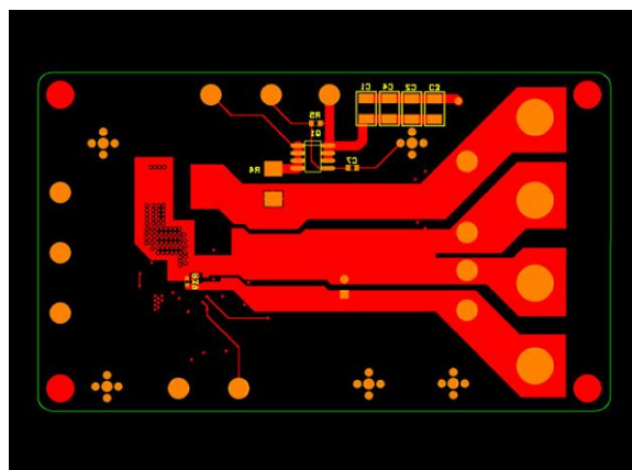
Fig. 17 - Bottom Layer
