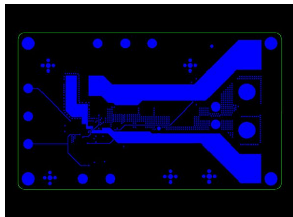
Fig. 15 - Mid Layer2
