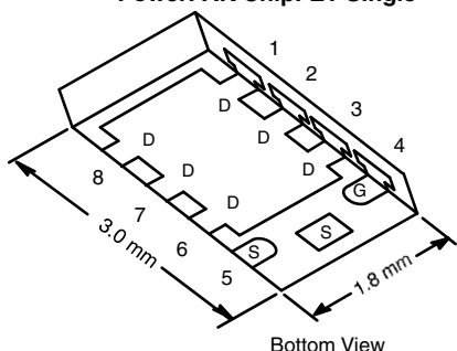
PowerPAK ChipFET Single
