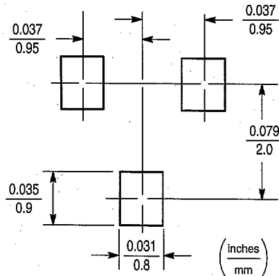
SOT-23
