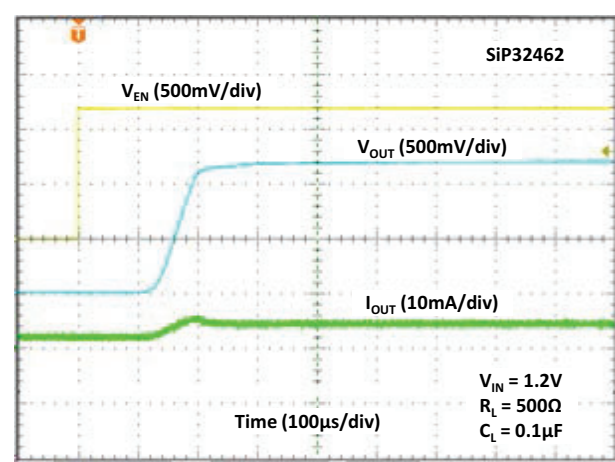
Fig. 30 - Turn-on Time
