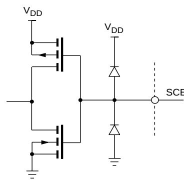
Fig. 3 Pin 14 SCE
