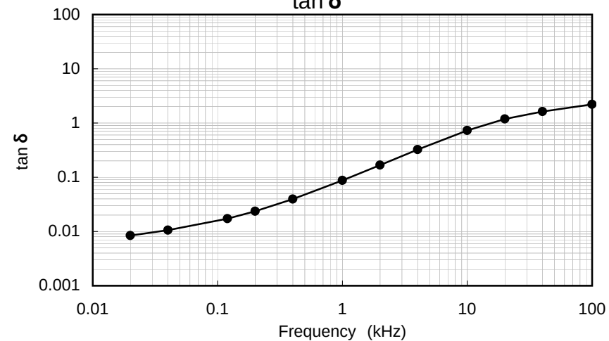
\tan \delta
