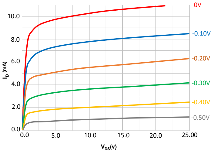
Figure 10. I_D vs. V_{DS} vs. V_{GS}
