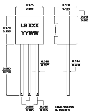
TO-92 3L
