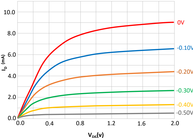
Figure 14. I_D vs. V_{DS} vs. V_{GS}
