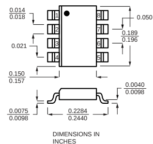
SOIC 8L
