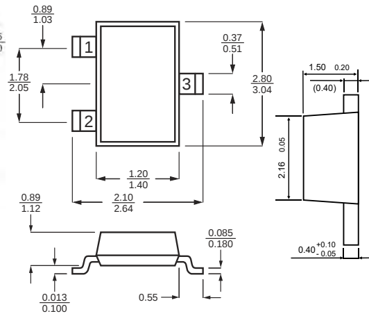
SOT-23
