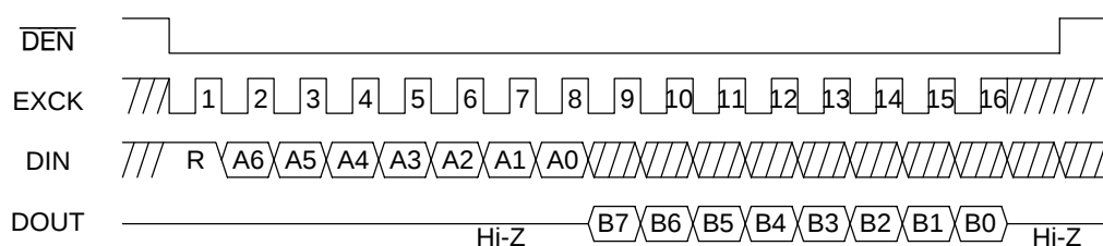
(d) Data Read Timing 2 (16-bit MCU)
