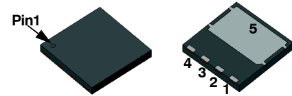
PQFN 8×8, 2P (Power88) CASE 483AP
