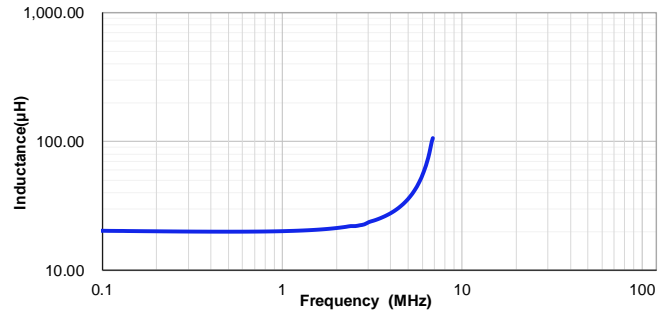
CSAD0880-220M
