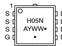
WDFN8 ( \mu 8FL) CASE 511AB
