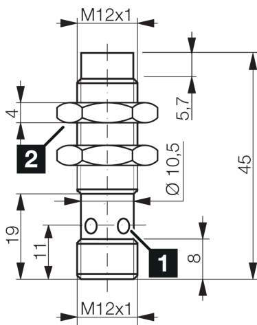
1) LED 4 x 90° (gelb) 2) Schlüsselweite 17 mm BN: braun BU: blau WH: weiß
