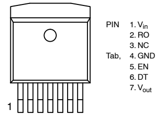
D2PAK-7
